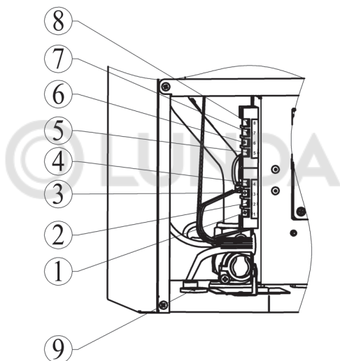
Рис. 11. Подключение дополнительных устройств
