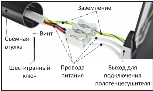
Схема 1. Подключение к проводам сети или к кабель-вилке
