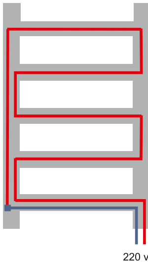
Схема протяжки нагревательного элемента.
