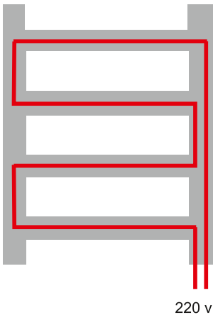
Схема протяжки нагревательного элемента.
