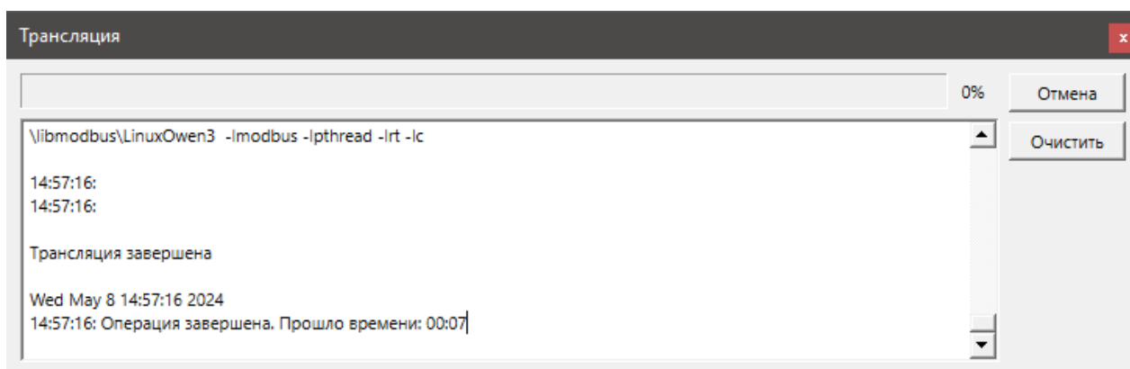
Рисунок 6.11 – Трансляция проекта
