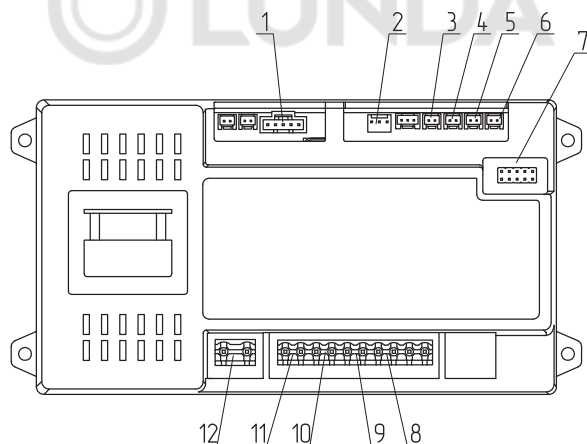
Рис.10 Подключение панели управления
