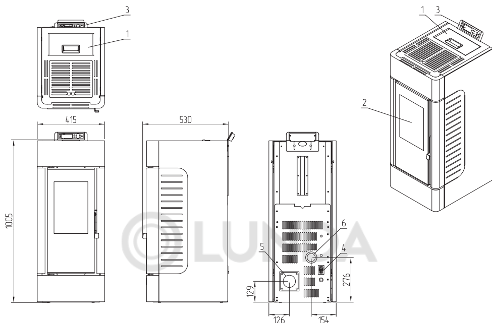
Рис.1 Устройство камина C12H21
