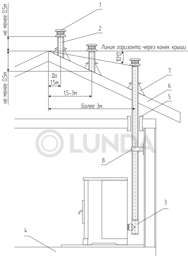
Рис.9 Подключение дымохода через крышу
