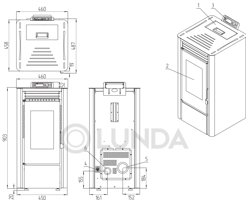
Рис.2 Устройство камина А9Н15
