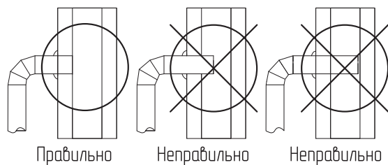
Рис.7 Подключение дымоотводящей трубы к кирпичному дымоходу
