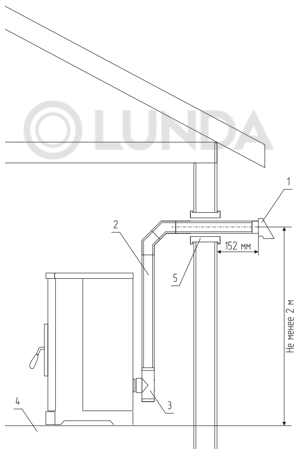
Рис.8 Подключение дымохода через стену
