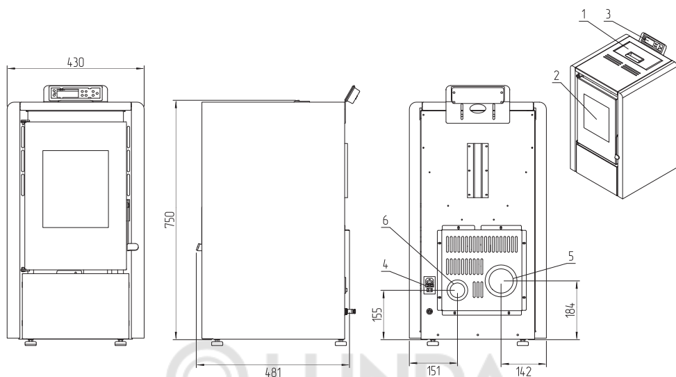
Рис.3 Устройство камина А6Н8
