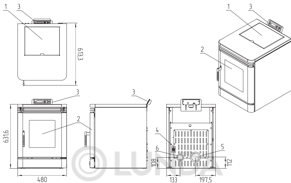
Рис.4 Устройство камина В6Н30
