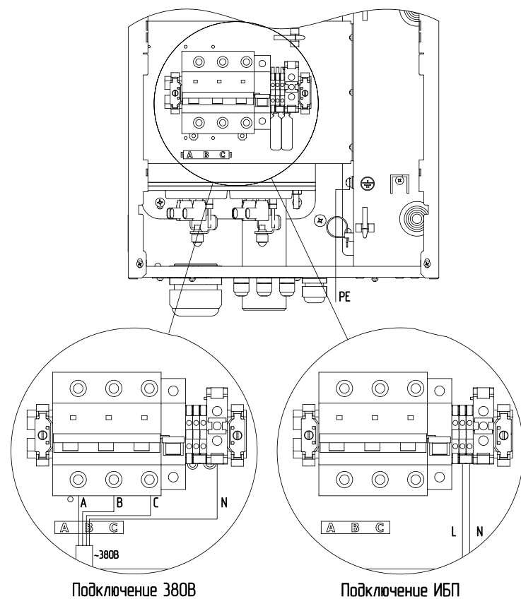
Рис.8 Схема подключения электрического котла ZOTA SOLID-X 30-60 кВт
