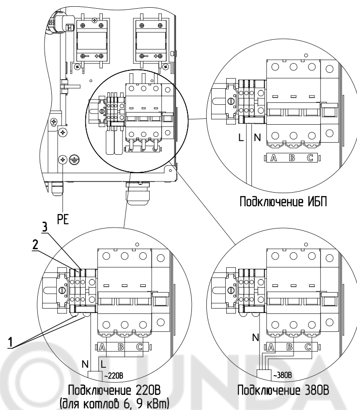
Рис.7 Схема подключения электрического котла ZOTA SOLID-X 6-24 кВт
