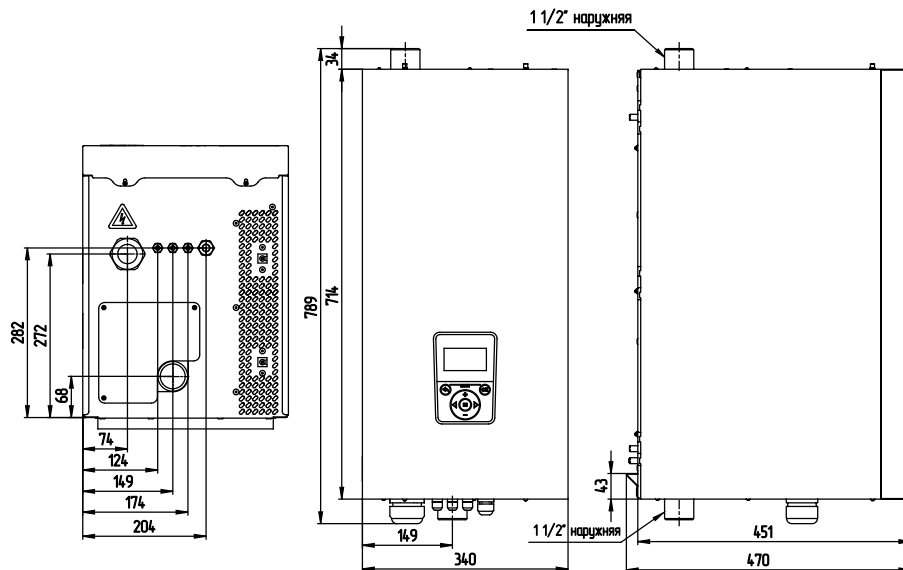
Рис.15 Габаритные размеры ZOTA SOLID-X 48-60 кВт
