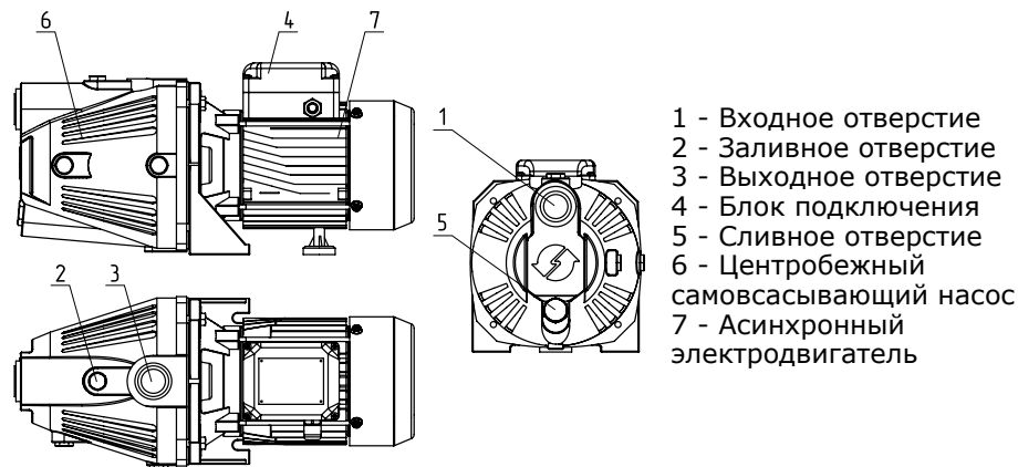
Рис.1. Конструкция насоса
