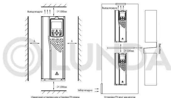
Рис. 3.1 Схема установки преобразователя частоты
