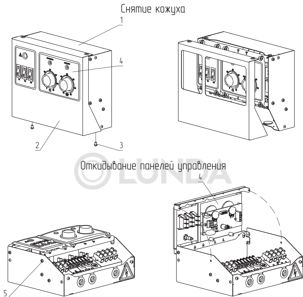
Рис.5 Конструкция кожуха, снятие, откидывание панелей управления
