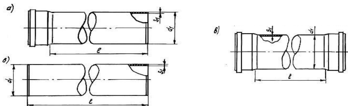
Рисунок 1. Конструкция и размеры труб
