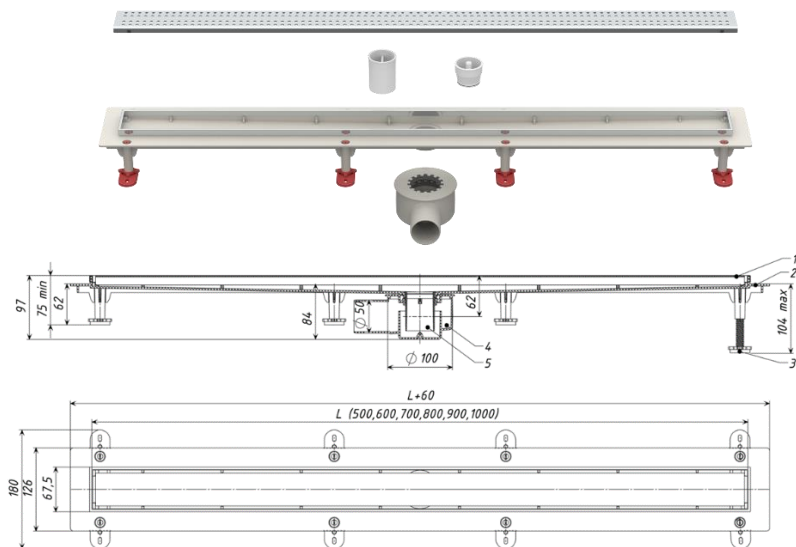
Рис. 1 – Габаритные размеры
