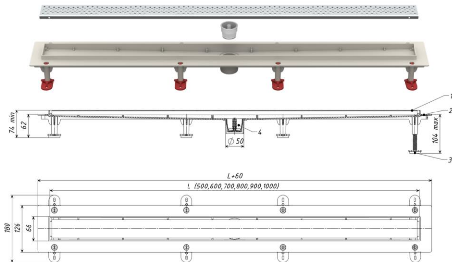
Рис. 1 – Габаритные размеры
