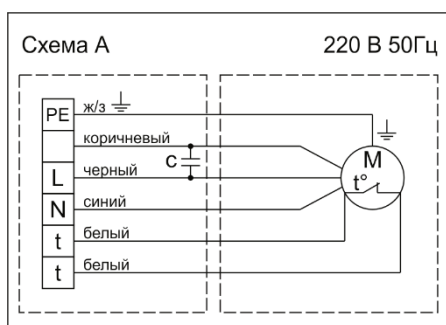
Рисунок 2. Схемы подключения вентилятора ВКП:
