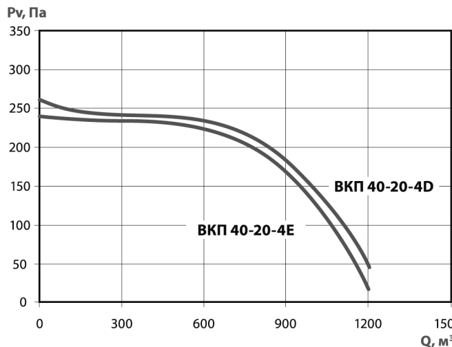
Рисунок 3. Аэродинамические характеристики вентиляторов канальных прямоугольных с вперед загнутыми лопатками (статическое давление от производительности)
