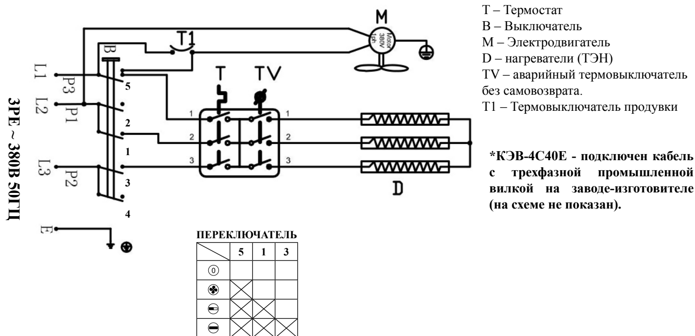
Рисунок 9. Электрическая схема тепловентиляторов КЭВ-4С40Е*, КЭВ-6С40Е и КЭВ-9С40Е
