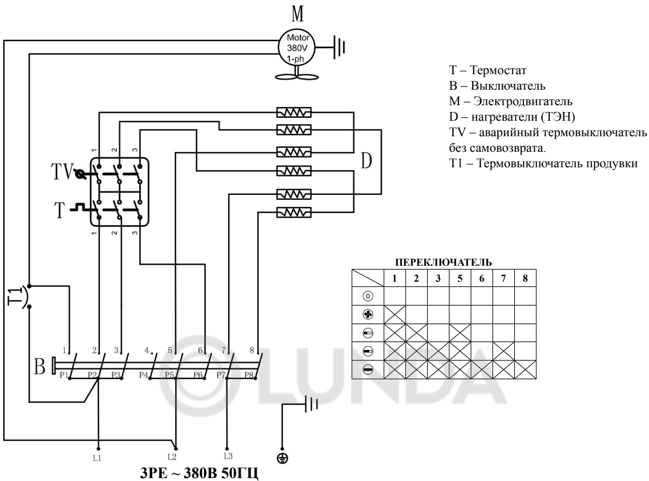
Рисунок 11. Электрическая схема тепловентилятора КЭВ-18С40Е
