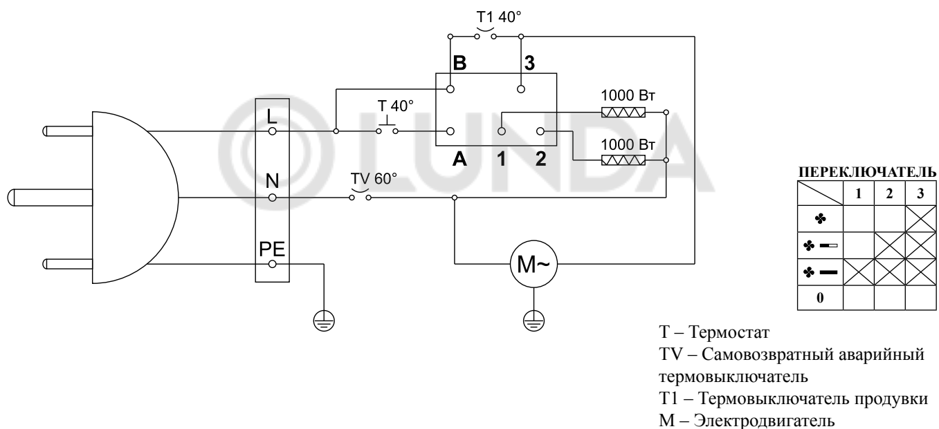
Рисунок 3. Электрическая схема тепловентилятора КЭВ-2С31Е
