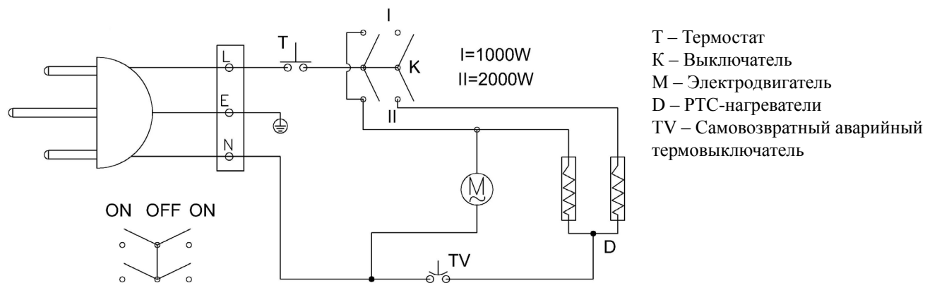
Рисунок 2. Электрическая схема тепловентилятора КЭВ-2С51Е
