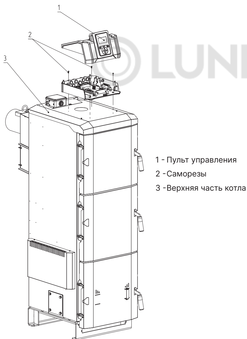
Рис.15 Установка пульта управления на котлы ZOTA Stahanov Black 16-65 кВт
