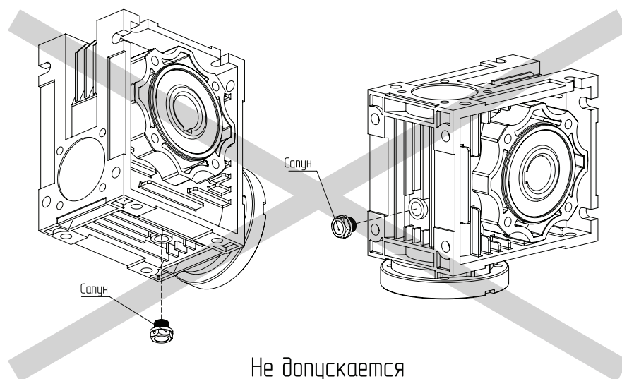
Рис.10 Установка сапунов
