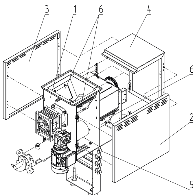
Рис.12 Схема монтажа съемных панелей механизма подачи (горелка условно не показана)
