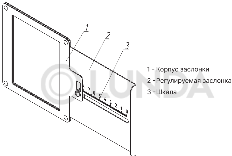
Рис.20 Заслонка вентилятора
