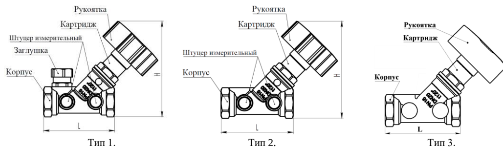
Рисунок 1. Клапан балансировочный ручной STAD.BY.
