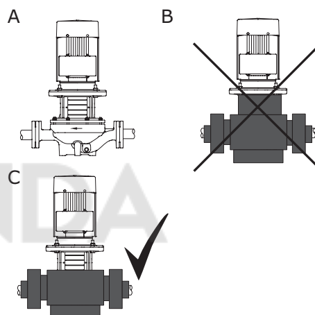
Рис. 12 Изоляция насосов TPE
