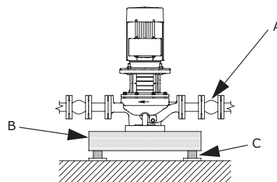
Рис. 10 Фундамент для насоса TPE
