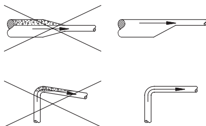
Рис. 9 Рекомендуемая конфигурация трубопроводов на стороне всасывания
