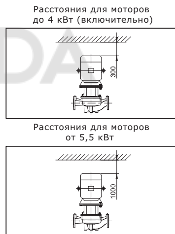
Рис. 8 Расстояния до стен/потолка для насосов TPE
