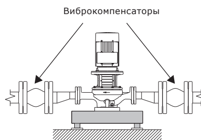
Рис. 11 Насос TPE с виброкомпенсаторами большего размера
