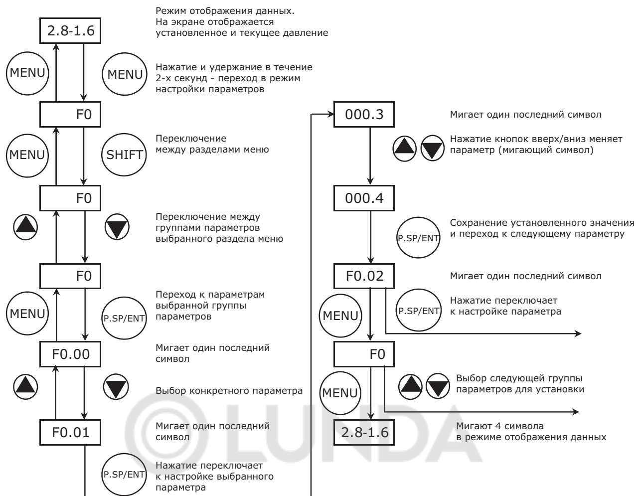
Рис. 20 Пример дерева настройки параметров
