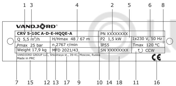
Рис. 2 Фирменная табличка
