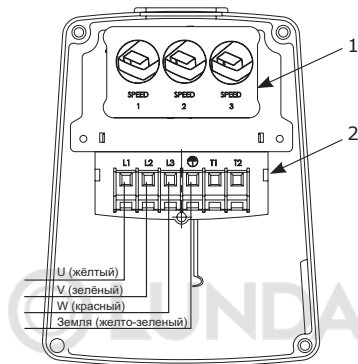
Рис. 6 Модуль переключения частоты вращения
