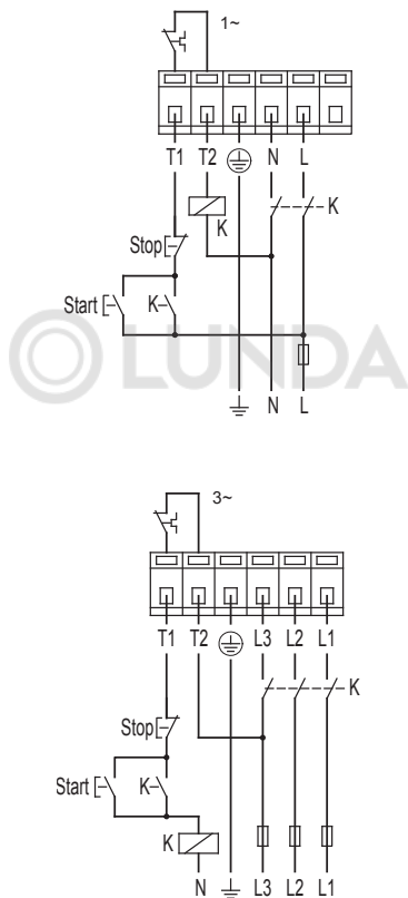
Рис. 8 Схема подключения при использовании внешнего электромагнитного пускателя ВКЛ/ВЫКЛ
