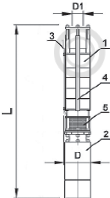
Рис. 1 Конструкция насоса
