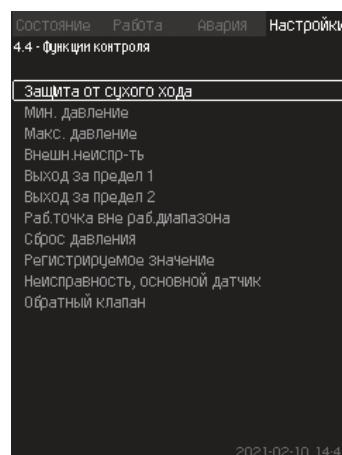
Рис. 103 Функции контроля
