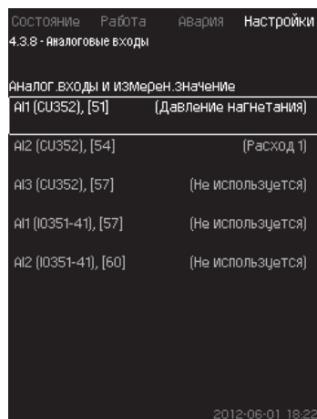
Рис. 80 Аналоговые входы
