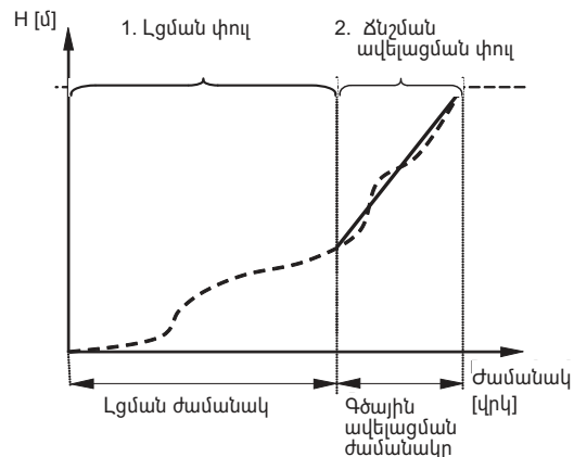
Նկար 76 Լցման և ճնշման ավելացման փուլեր
