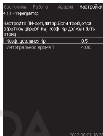
Рис. 42 ПИ-регулятор
