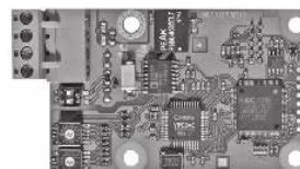
Рис. 139 Модуль передачи данных Grundfos CIM
