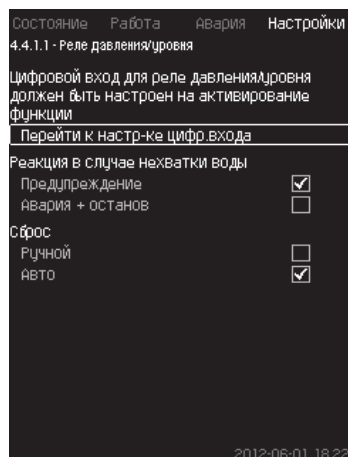
Рис. 105 Реле давления/уровня
