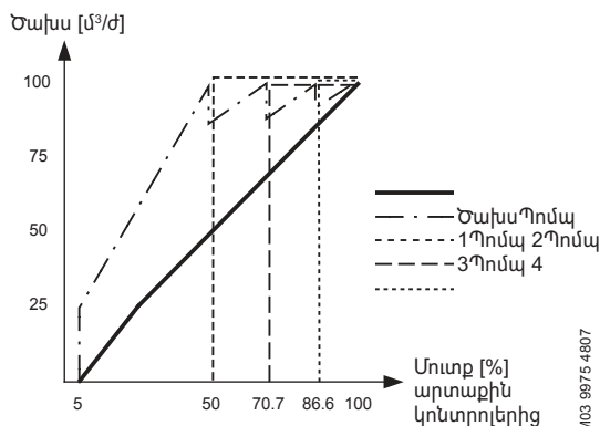
Նկար 30 Կարգավորման բնութագիր MPC-F-ի համար անջատված կոնտուրում
