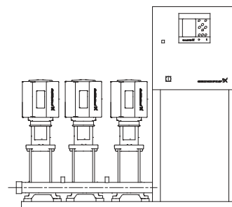
Рис. 25 Установка, регулируемая встроенным ПИ-регулятором (замкнутый контур)
