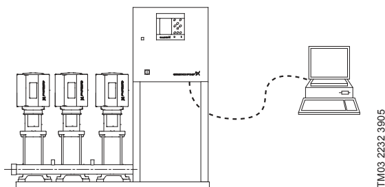
27-сур. Тышкы көзөмөлдөгүч менен басымды жогорулатуу орнотмосу (ачык чөйрөсиздик)
