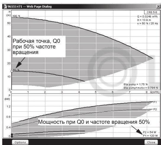
Рис. 95 Показание мощности при Q_0 и 50 % частоте вращения
