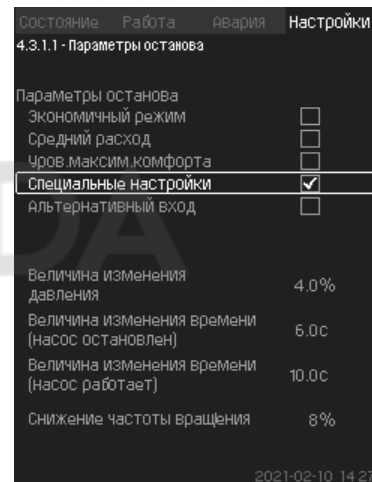
Նկար 73 Հատուկ կարգավորումներ
