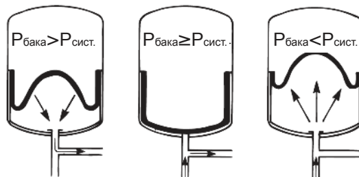
Рис. 5 Мембранный напорный бак (P - давление)
