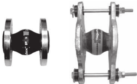
Նկար 8 Թրթռաներդիրներ ռեզինե միջադիրներով՝ առանց սահմանափակիչ առձգիչների և դրանցով
