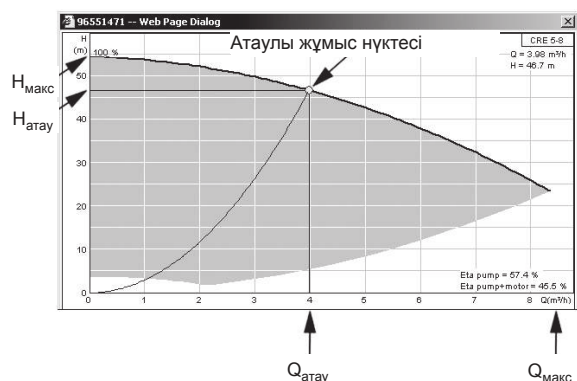
93-сур. Көрсеткіш Q_{атау} , H_{атау} , H_{макс} және Q_{макс}
