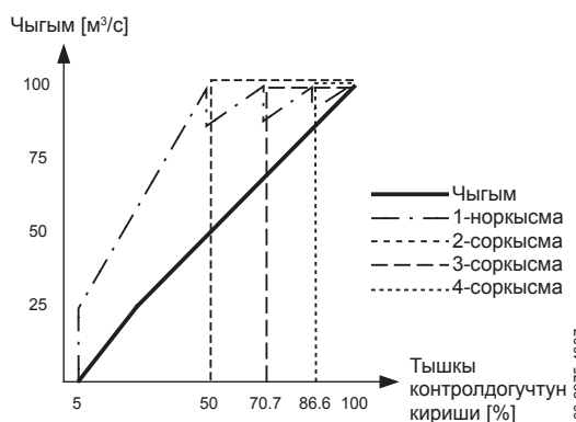
30-сур. MPC-F үчүн ачык чөйрөсиздик үчүн жөнгө салуучу мүнөздөмө
