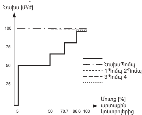
Նկար 31 Կարգավորման բնութագիր MPC-S-ի համար անջատված կոնտուրում
