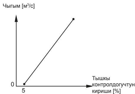
27-сур. Тышкы көзөмөлдөгүч менен басымды жогорулатуу орнотмосу (ачык чөйрөсиздик)
