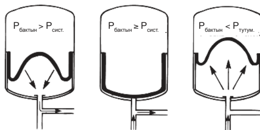
5-сүр. Мембраналык оргутуучу бак (P-басым)
