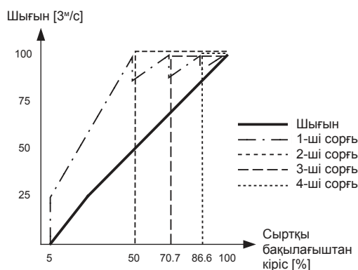
30-сур. MPC-F үшін алшақталған контурда реттелуші сипаттама
