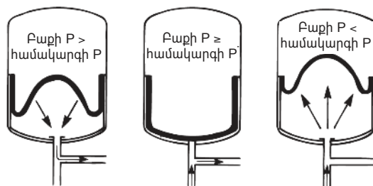
Նկար 5 Թաղանթային ձնշումային բաք (P՝ ձնշում)
