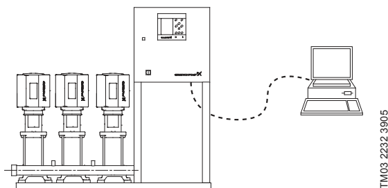
27-сур. Сыртқы бақылағышпен қысымды арттыру қондырғысы (алшақталған контур)
