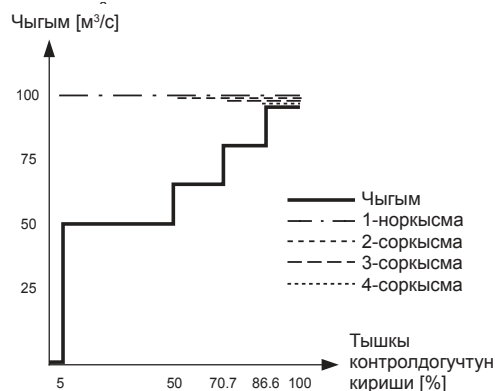
31-сур. MPC-S үчүн ачык чөйрөсиздик үчүн жөнгө салуучу мүнөздөмө
