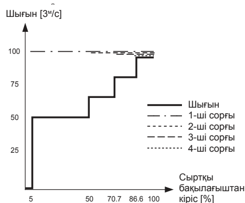
31-сур. MPC-S үшін алшақталған контурда реттелуші сипаттама
