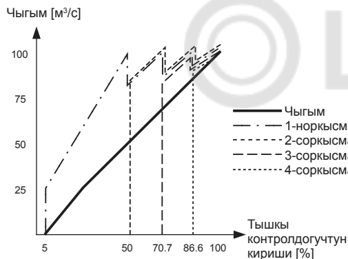
29-сур. MPC-E үчүн ачык чөйрөсиздик үчүн жөнгө салуучу мүнөздөмө
