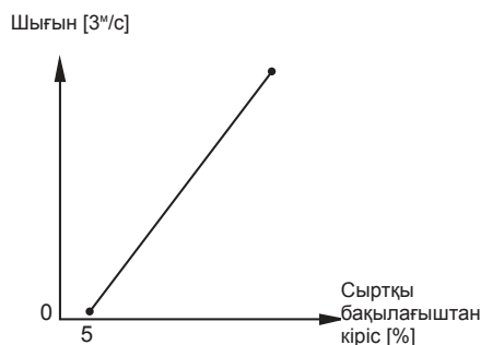
28-сур. Алшақталған контур үшін реттелуші сипаттама
