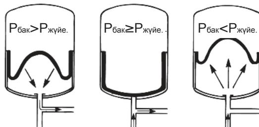
5-сур. Мембраналы арынды бак (P – қысым)
