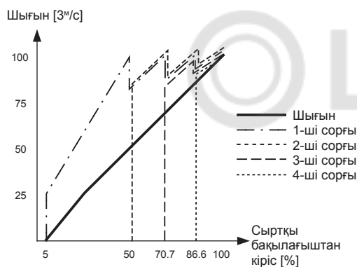
29-сур. MPC-E үшін алшақталған контурда реттелуші сипаттама
