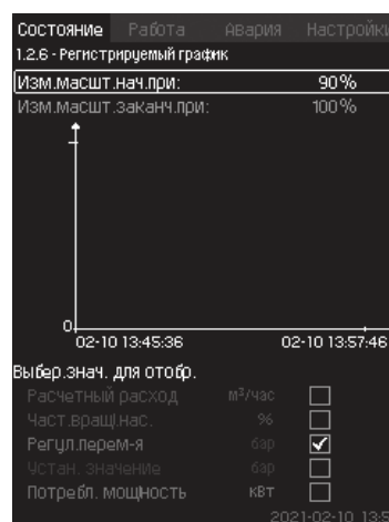
Рис. 19 Регистрируемый график
