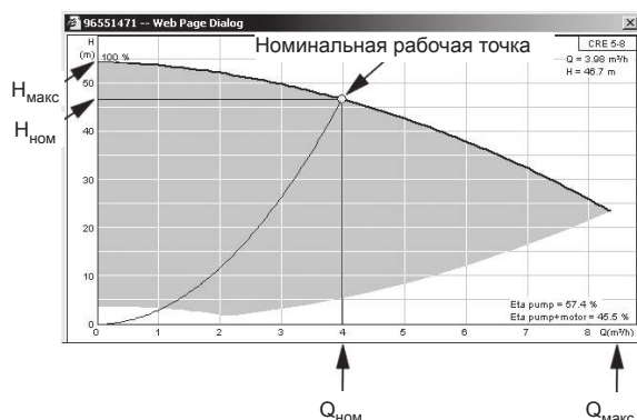
Рис. 93 Показание Q НОМ , H НОМ , H МАКС и Q МАКС
