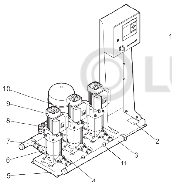
1-сур. Hydro MPC қысымды арттыру қондырғысы
