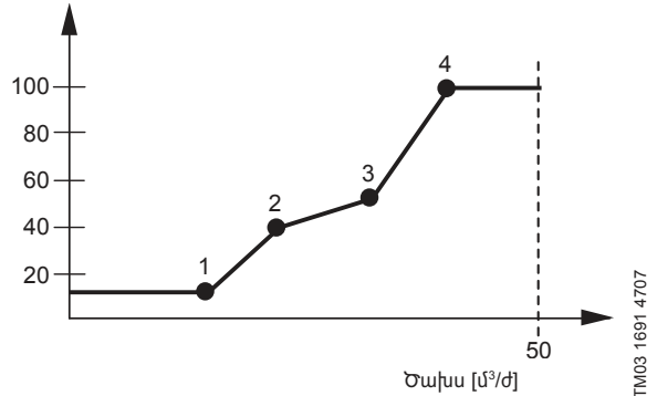
Նկար 47 Նշանակված արժեքի նկատմամբ ազդեցության և փախսի միջև հարաբերակցությունը
