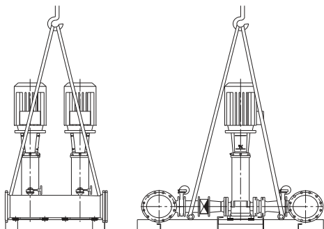
4-сур. Hydro MPC дұрыс көтеру
