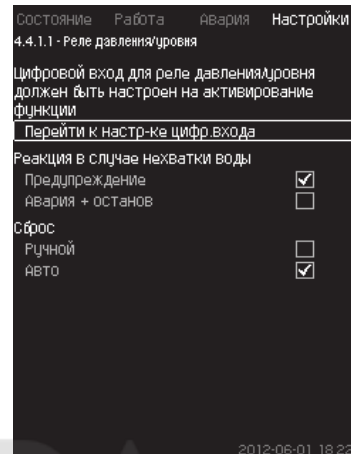
105-сур. Қысым/деңгей релесі
