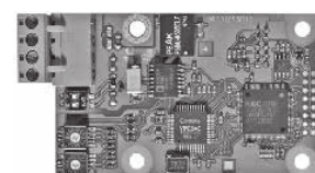
Նկար 139 Grundfos CIM տվյալների փոխանցման մոդուլ
