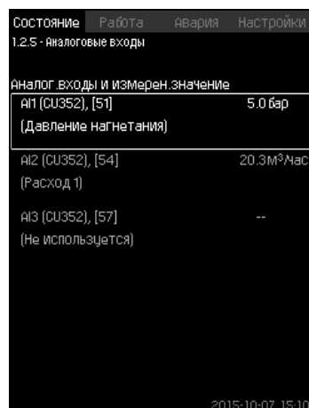
Рис. 13 Аналоговые входы
