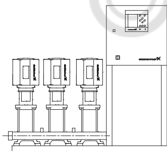
Рис. 20 Установка, регулируемая встроенным ПИ-регулятором (замкнутый контур)
