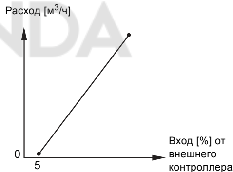
Рис. 23 Регулировочная характеристика для разомкнутого контура
