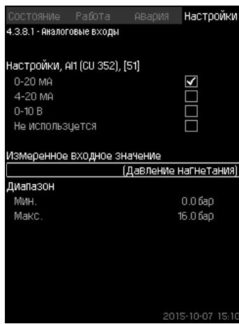
Рис. 75 Аналоговые входы
