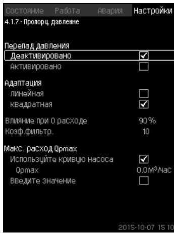
Рис. 47 Пропорц. давление
