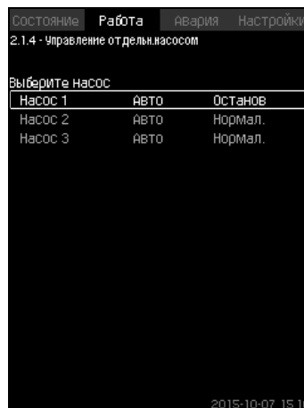
Рис. 28 Управление отдельн.насосом
