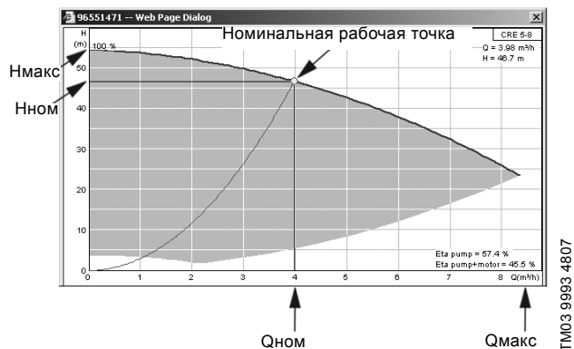
Рис. 86 Показание Q_{ном} , H_{ном} , H_{макс} и Q_{макс} (WebCAPS)
