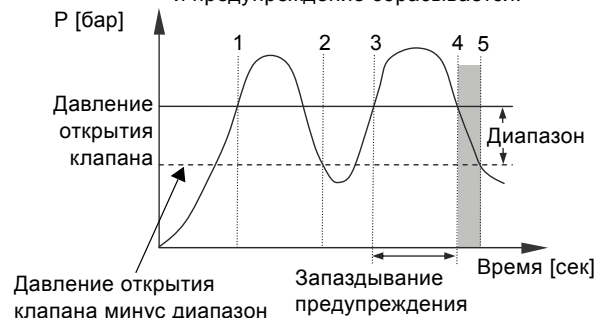
Рис. 105 Сброс давления
