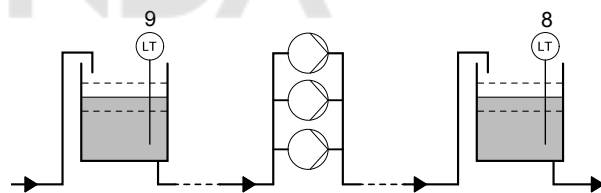
Рис. 127 Контроль уровня
