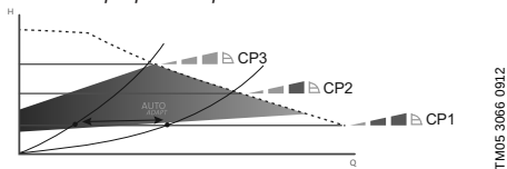
Рис. 19 Три кривые/настройки регулирования с постоянным давлением
