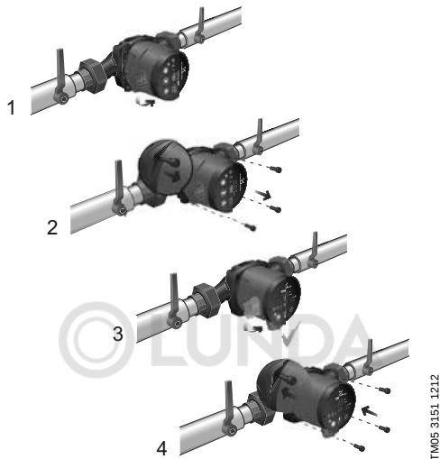
Рис. 7 Изменение расположения блока управления
