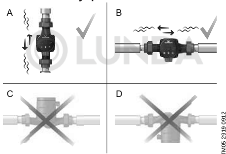
Рис. 4 Положение блока управления
