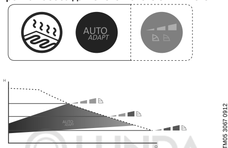
Рис. 20 Выбор настроек насоса в соответствии с типом системы
