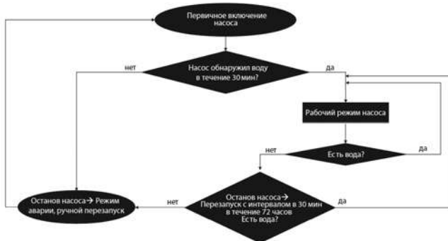
Рис. 25 Алгоритм работы защиты от «сухого» хода
