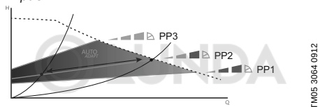
Рис. 17 Три кривые/настройки пропорционального регулирования
