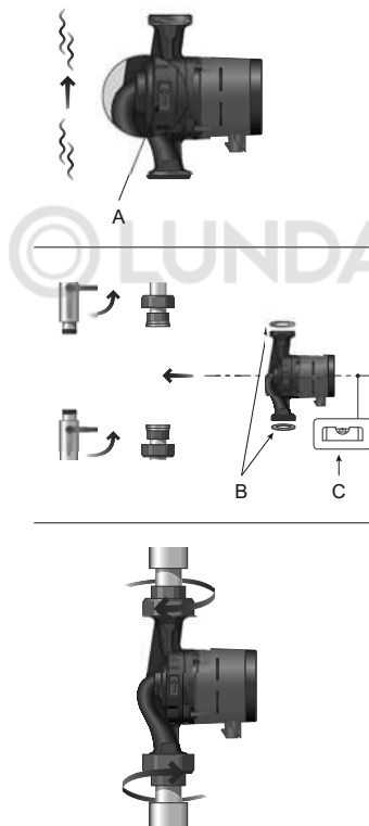
Рис. 3 Монтаж насоса ALPHA2
