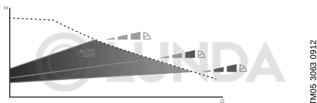
Рис. 16 Выбор настроек насоса в соответствии с типом системы
