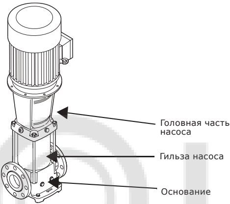
Рис. 9 Горячие поверхности на насосе CRV-C/CRV-HP
