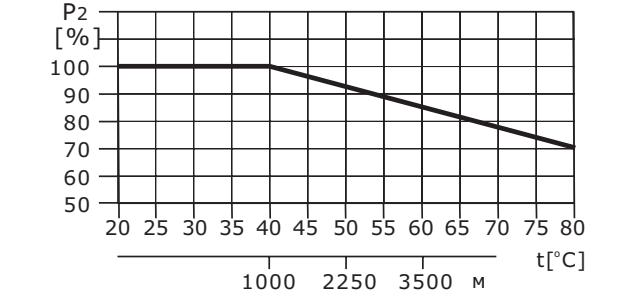
Рис. 18 Мощность электродвигателя в зависимости от температуры/высоты над уровнем моря
