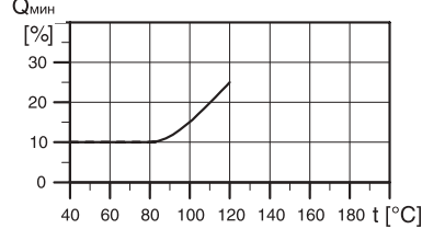
Рис. 20 Минимальная подача
