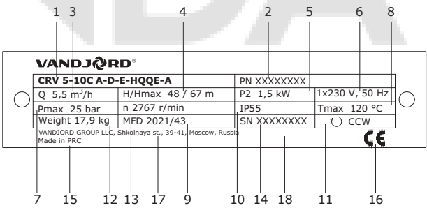
Рис. 2 Фирменная табличка
