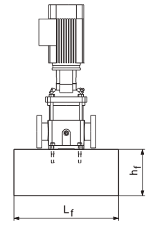
Рис. 4 Правильный монтаж
