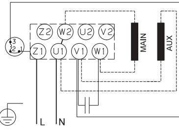
Рис. 13 Подключение «высокого напряжения», 0,37 - 0,75 кВт
