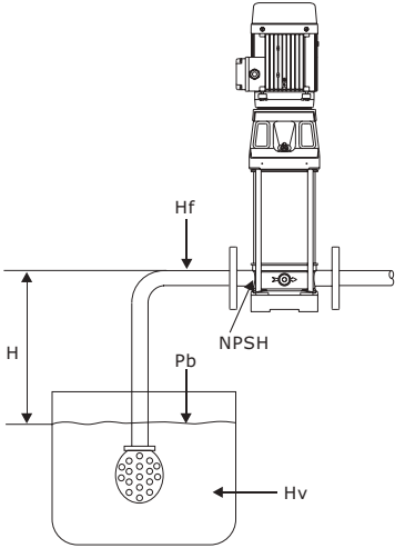
Рис. 19 Открытая система с насосом серии CRV-C/CRV-HP
