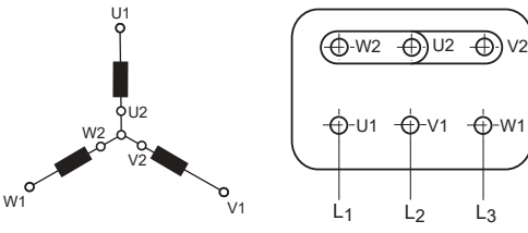
Рис. 11 Соединение звездой
