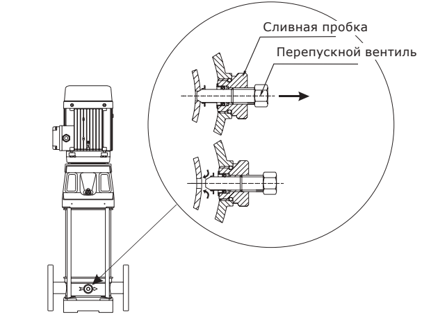
Рис. 17 Пробка сливного отверстия с перепускным вентилем
