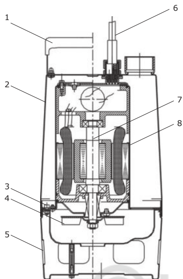
Рис. 10 Чертеж в разрезе APV.40 V
