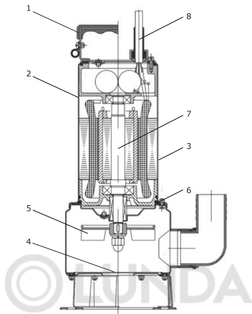
Рис. 9 Чертеж в разрезе APV.40B/45B/50B V
