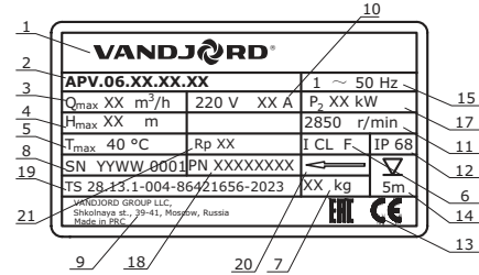
Рис. 5 Фирменная табличка насосов серии APV
