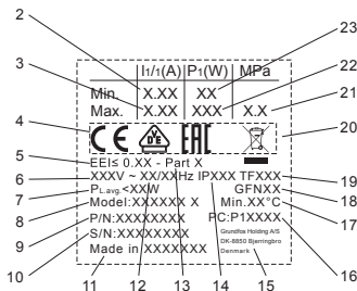
2-сур. ALPHA SOLAR фирмалық тақтайшасы
