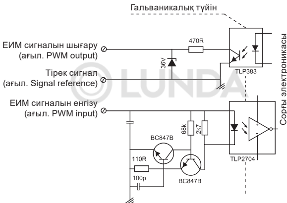
18-сур. Сорғы интерфейсінң электрлі сызбасы
