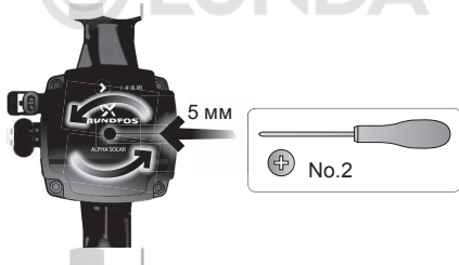
19-сур. Сорғы білігін бұғаттан шығару
