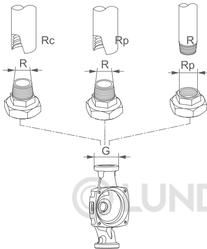
Սկար 20 Պարուրակային միացումների տեսակները
