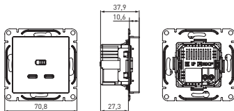
Рис. 5 Механизм розетки 2USB-C UP1-S0*-2USBC
