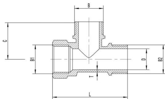
Тройник, ВР-НР-НР
