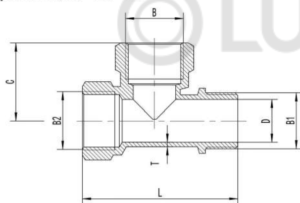
Тройник, ВР-ВР-НР
