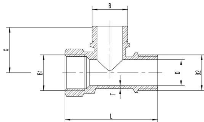
Тройник, ВР-НР-НР
