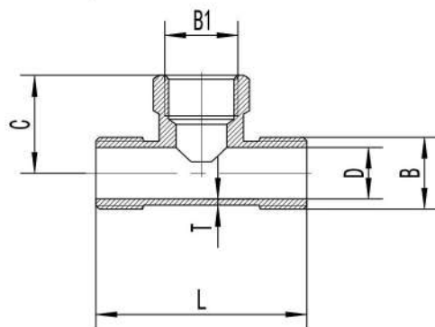
Тройник, НР-ВР-НР
