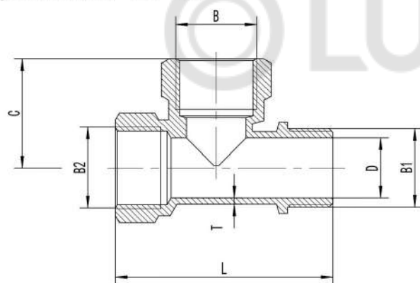
Тройник, ВР-ВР-НР
