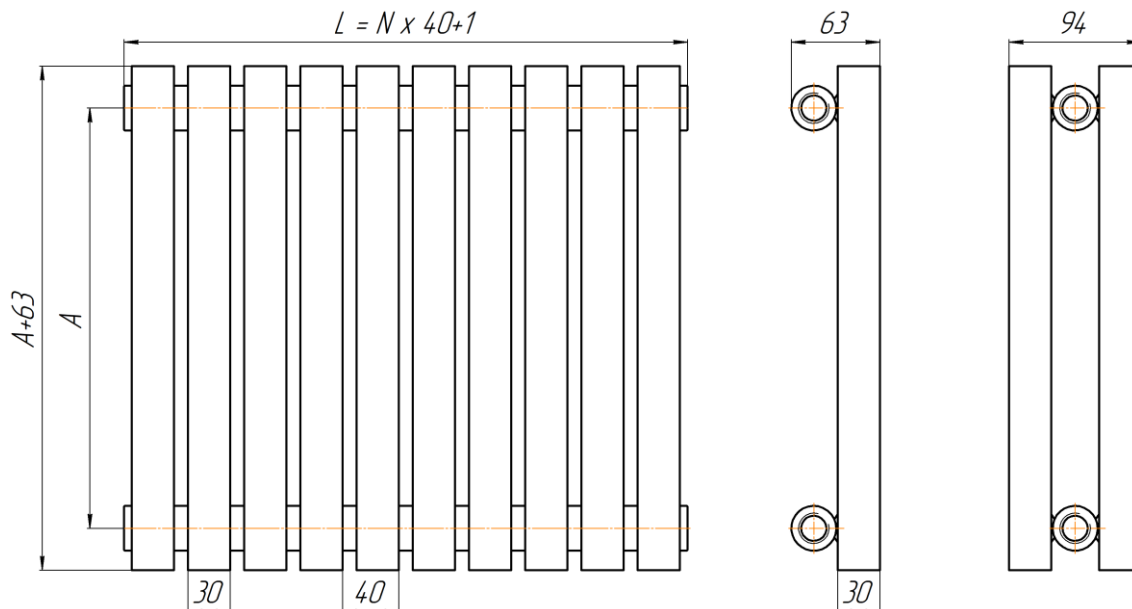
Рис 1. Радиатор «QUADRUM 30 V», где: А – межцентровый (монтажный) размер, мм; N – количество секций; L – габаритная длина, мм;
