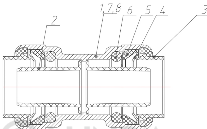
Рисунок 1. Разрез пуш-фитинга
