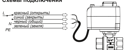
Электрическая схема подключения крана с электроприводом серии Neptun Bugatti Click 230B (рис. 3)
