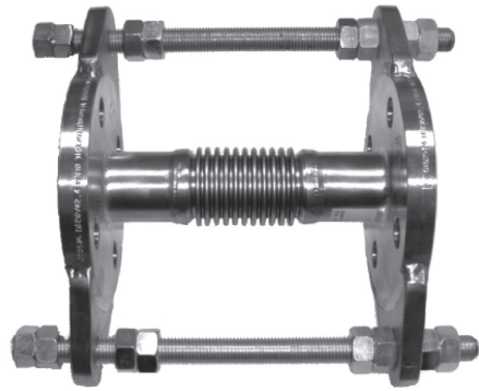
Рис. 18 Вибровставка с металлическим сальфоном и ограничительными стяжками
