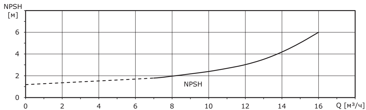
Рис. 14 Кривая NPSH для VCM 12
