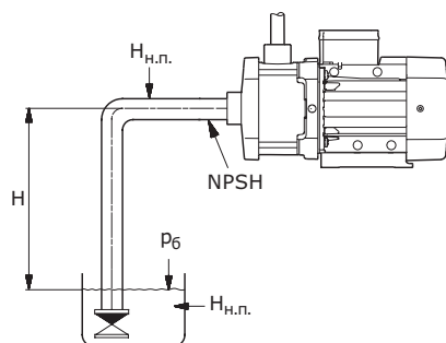
Рис. 9 Минимальное давление на входе
