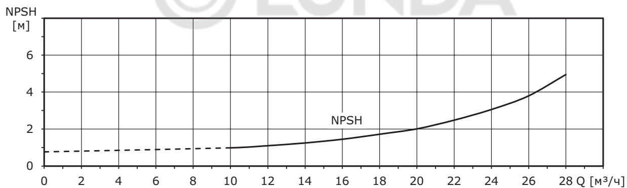
Рис. 16 Кривая NPSH для VCM 20
