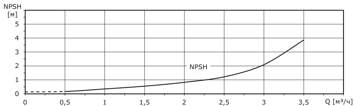
Рис. 11 Кривая NPSH для VCM 2
