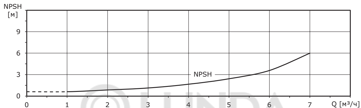
Рис. 12 Кривая NPSH для VCM 4
