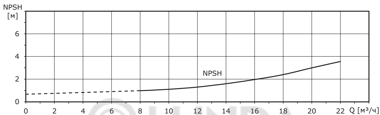
Рис. 15 Кривая NPSH для VCM 15
