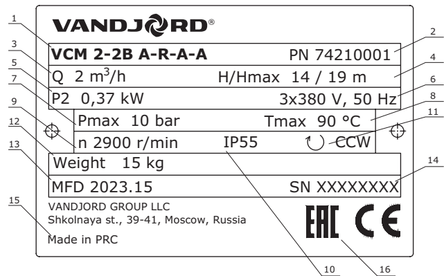
Рис. 2 Фирменные таблички насоса
