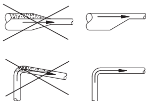
Рис. 4 Трубопровод
