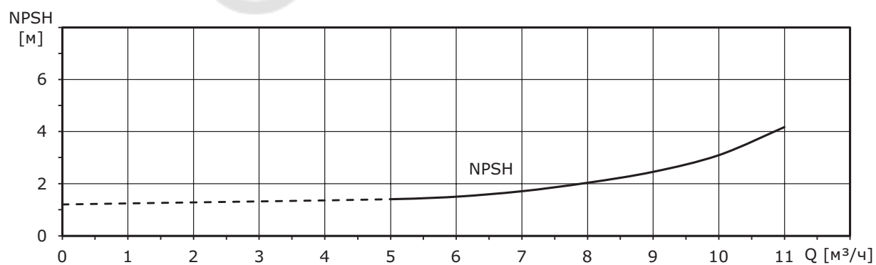
Рис. 13 Кривая NPSH для VCM 8
