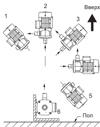
Рис. 3 Положения насоса
