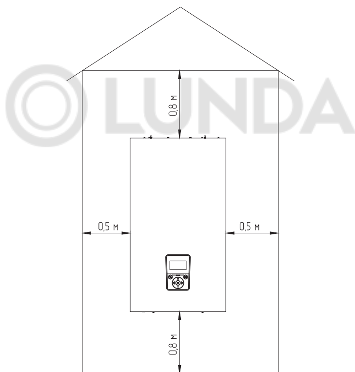
Рис. 7 Схема размещения котла в котельной
