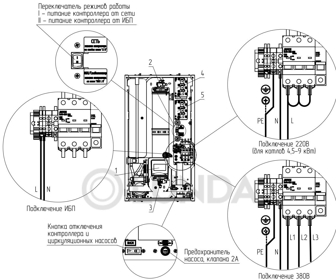
Рис. 5 Схема подключения и органы управления электрического котла ZOTA МК-X V2 от 4,5 до 24 кВт
