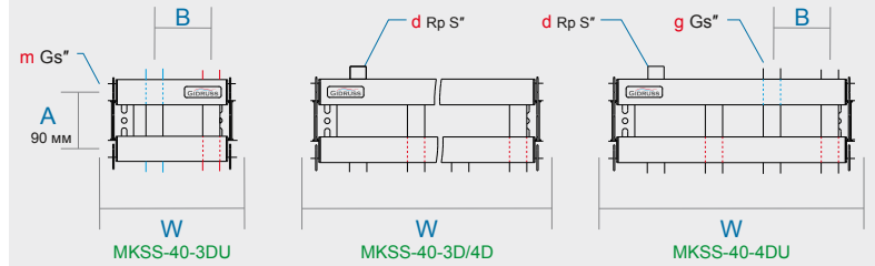
Рис.2. Габаритные размеры серии MK/MKSS-60/100
