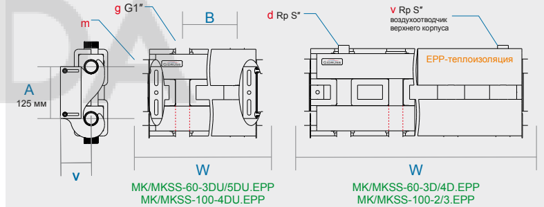
Рис.3. Габаритные размеры серии MK/MKSS-150
