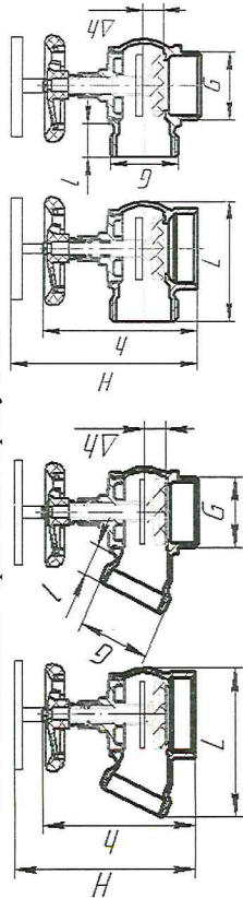
Исполнение 1: КПДМ, КПЧ, КПК. Исполнение 2: КПДМ, КПЧМ, КПКМ, КПКМ, КПКМ
