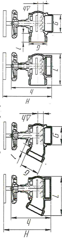
Рисунок 1—Внешний вид клапанов угловых моделей КПЛ, КПЧ, КПК и КПЛМ, КПЧМ, КПКМ
