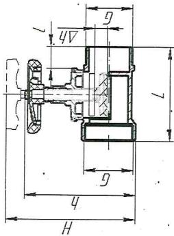
Рисунок 2 – Внешний вид прямой модели КЛПМ, КЛЧП и КПКП.
