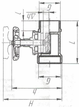
Рисунок 1 – Внешний вид клапанов угловых моделей КЛЛ, КЛЧ, КПК и КПКМ, КПКМ, КПКМ
